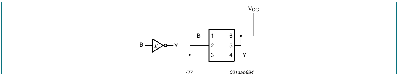
Fig. 11. Inverter
