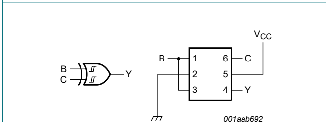
Fig. 9. 2-input XOR gate
