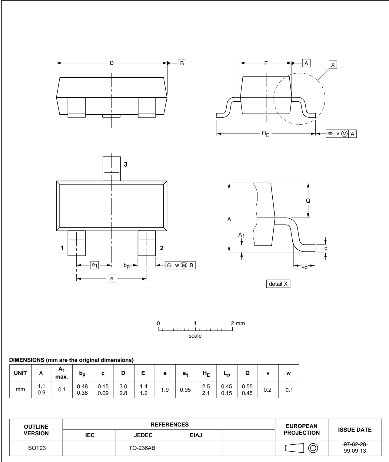
Fig 15. SOT23.
