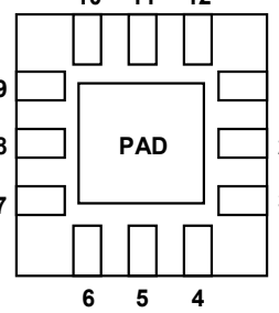
NJM2904CME2 (Note1, 2, 3)
