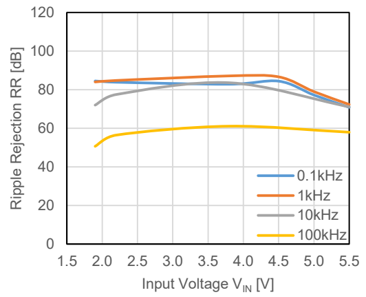
RP122x28xx, I OUT = 250 mA
