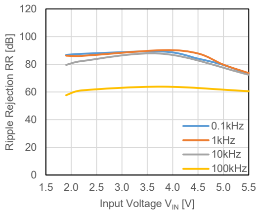
RP122x28xx, I OUT = 100 mA
