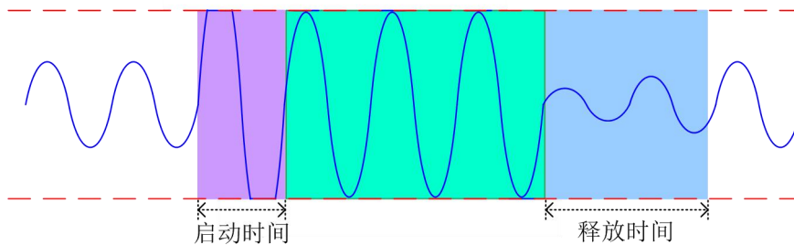
图 7 防失真工作模式下的音频输出信号
