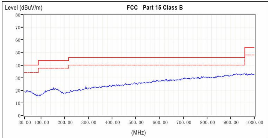
图 1 EMI 测试频谱图
