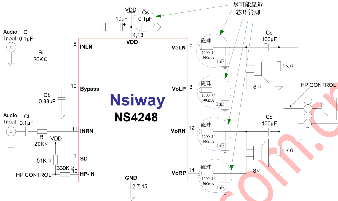
图 2 NS4248 加磁珠应用电路
