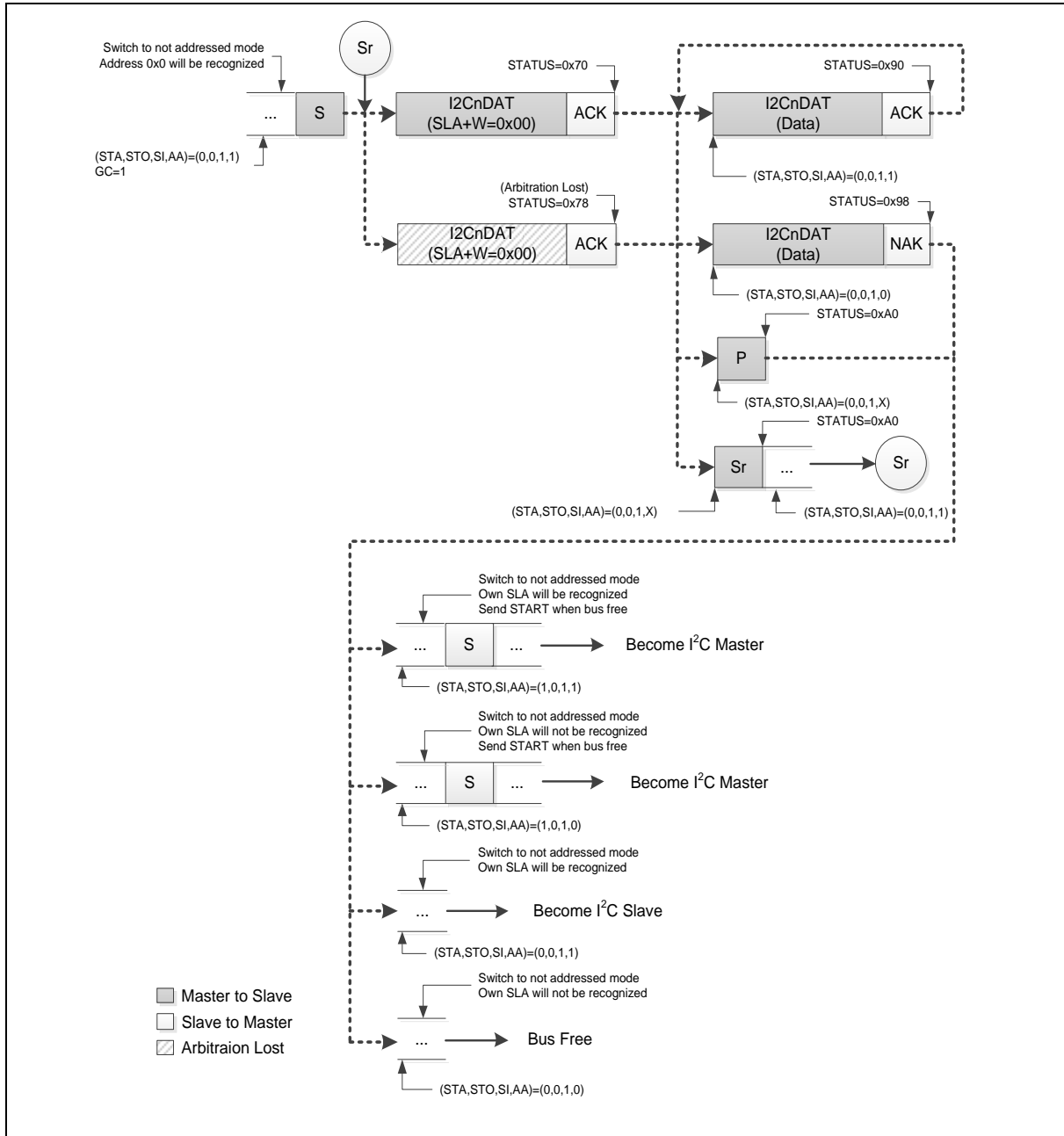
图 6.11-13 广播呼叫模式流程和状态
