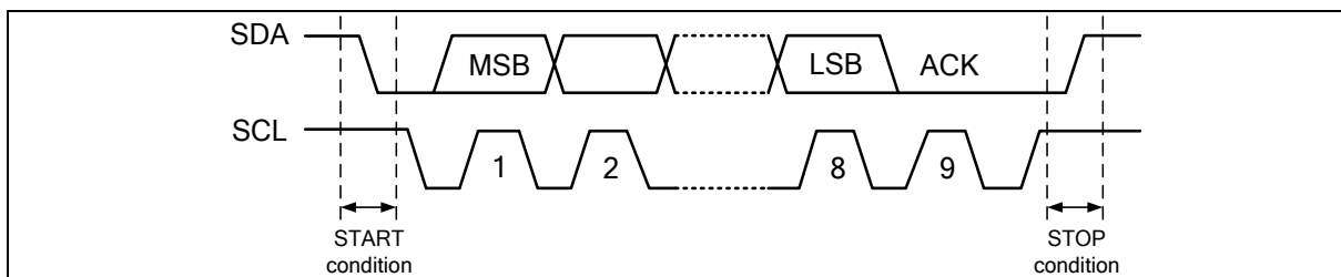
图 6.11-2 I 2 C 总线协议
