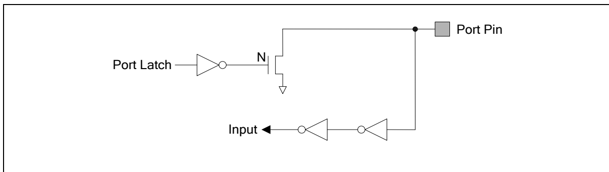
图 6.4-4 开漏模式
