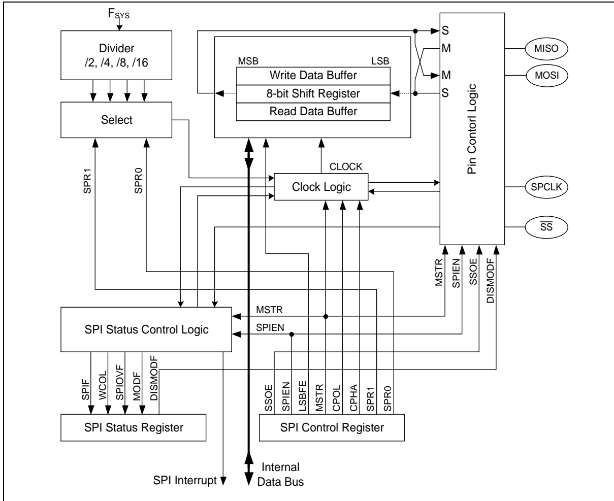
图 6.12-1 SPI 框图
