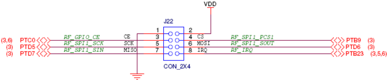
Figure 16. Optional add-on 2.4 GHz RF module
