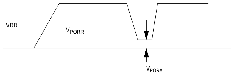
Figure 13 POR Re-arm
