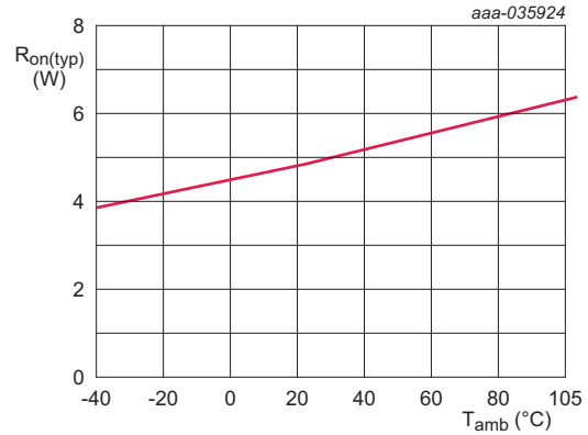
b. I_O = 15 mA; V_I = 2.4 V; V_{I(EN)} = 4.5 V
