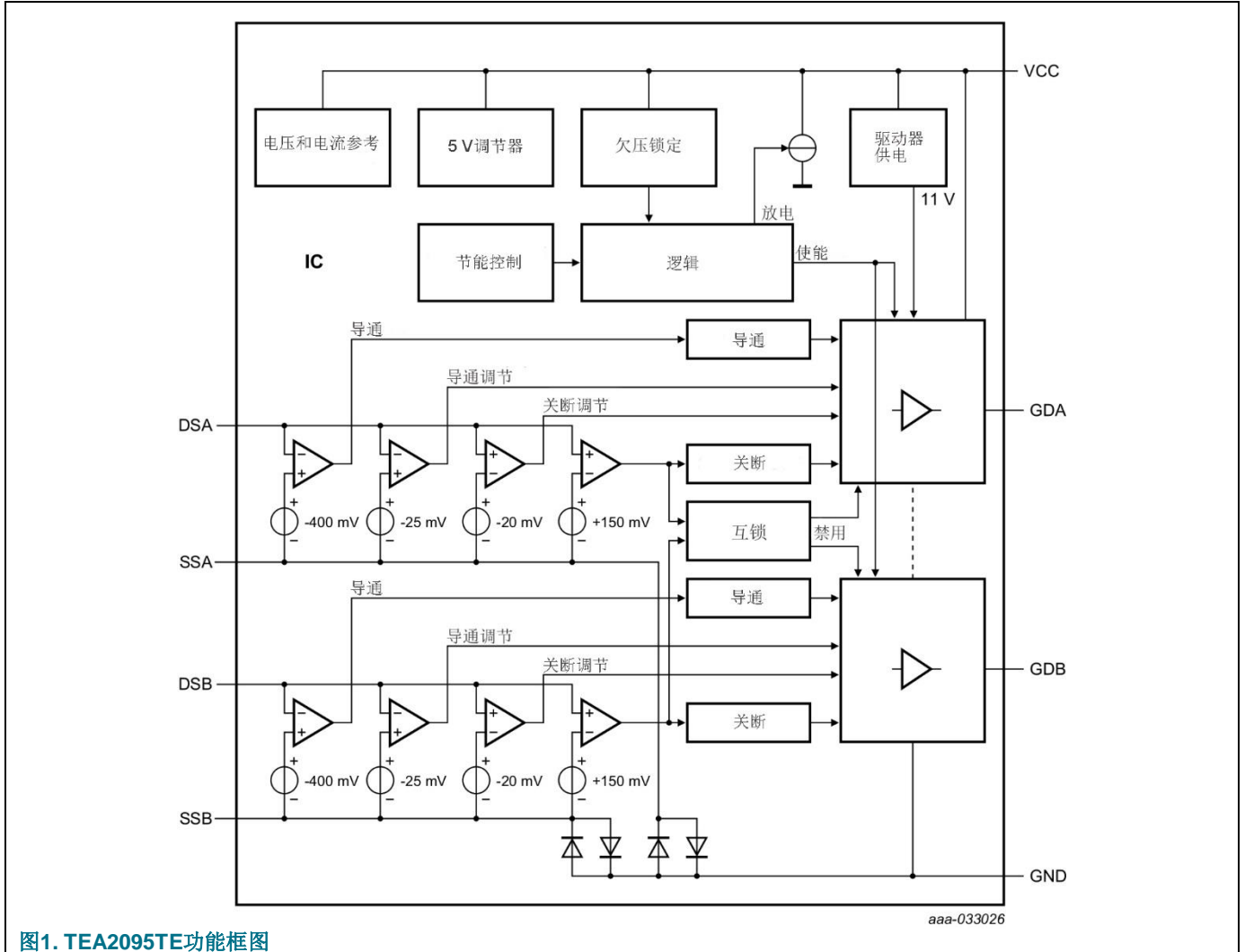
图1. TEA2095TE功能框图
