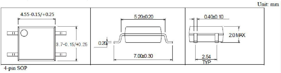
外形尺寸
