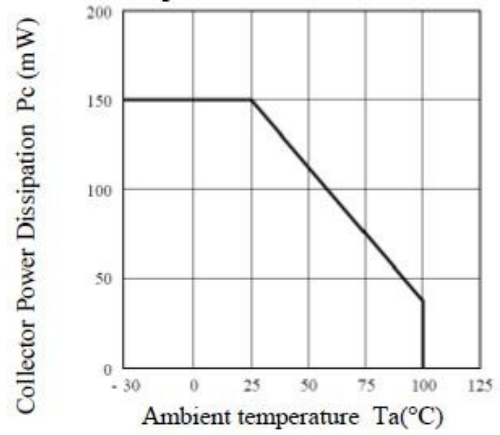
图 2: 集电极功耗 VS 温度
