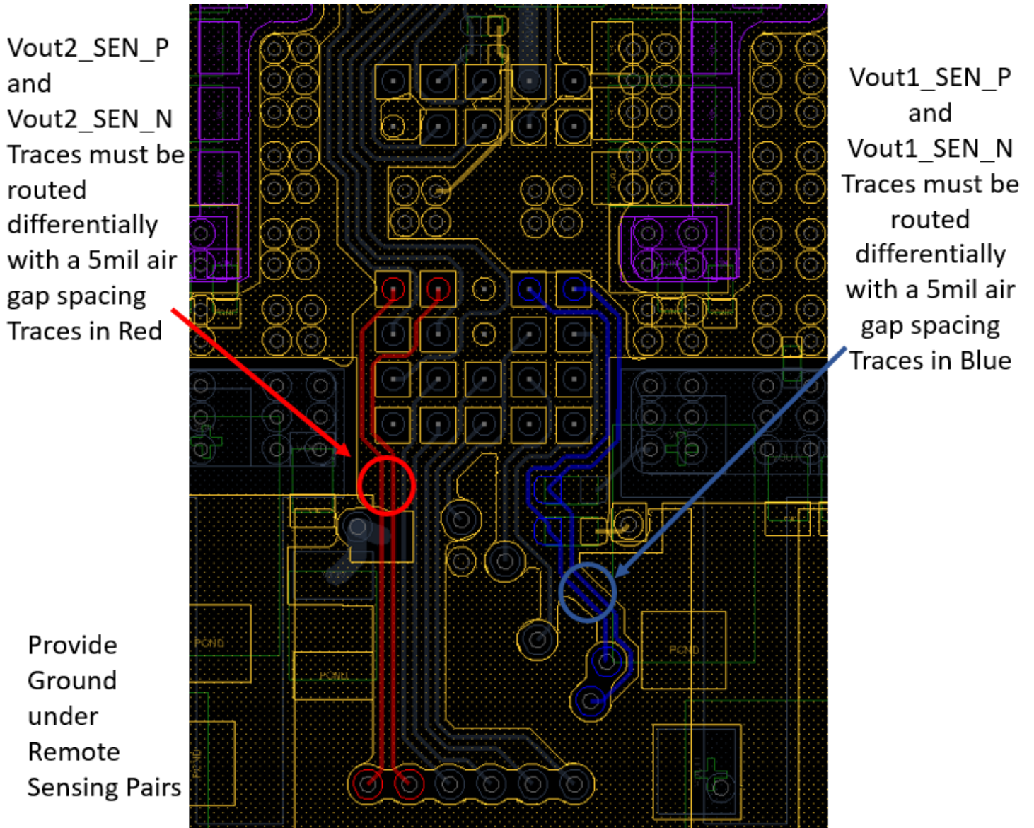
Figure 33 : VSense Traces
