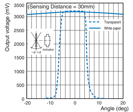
B5W-LB2101
