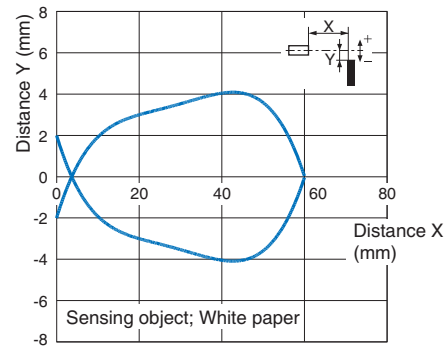
B5W-LB2
