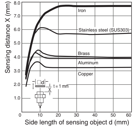
E2A-S18□S08
