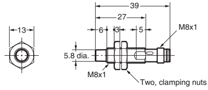
E2A-S08KN04-M5-□□/ E2A-S08KN04-M3-□
