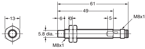
E2A-S08LN04-M5-□□/ E2A-S08LN04-M3-□
