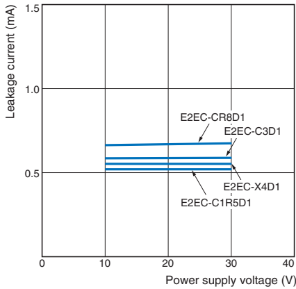
E2EC
