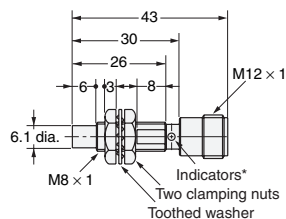
Diagram 19 E2E-X4MD□-M1(G) E2E-X2ME□-M1/E2E-X2MF□-M1
