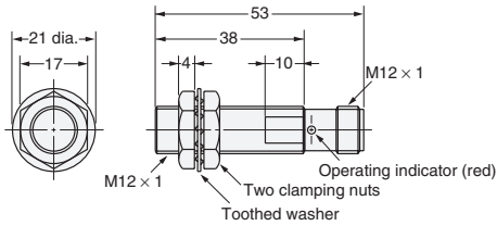
Fig. 24: E2E-X7D□-M1(G)/E2E-X5E□-M1/F□-M1 E2E-X5Y□-M1
