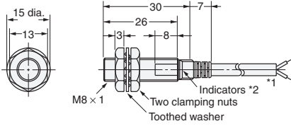
Diagram 1 E2E-X2D□ E2E-X1R5E□/F□
