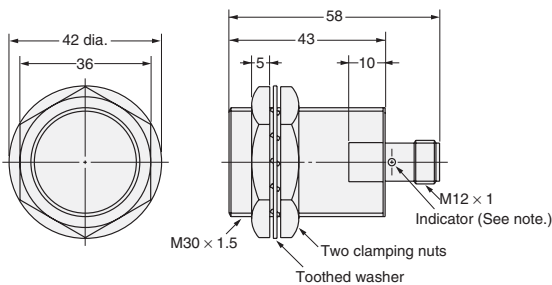
Fig. 25 : E2E-X10D□-M1(G)/E2E-X10E□-M1/F□-M1 E2E-X10Y□-M1
