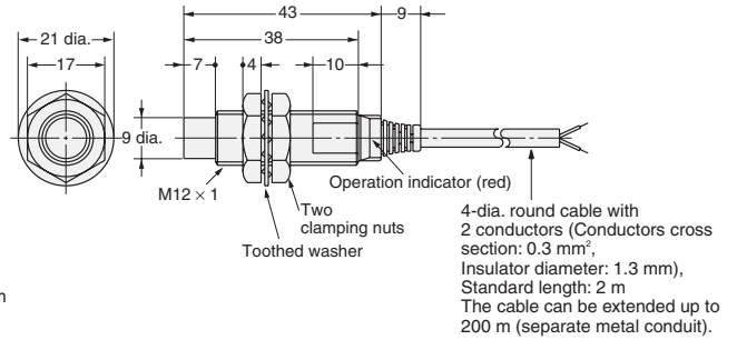
Fig. 11 : E2E-X5MY□
