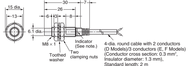
Fig. 5 : E2E-X4MD□ E2E-X2ME□/F□
