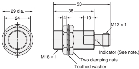
Fig. 23 : E2E-X7D□-M1(G)/E2E-X5E□-M1/F□-M1 E2E-X5Y□-M1
