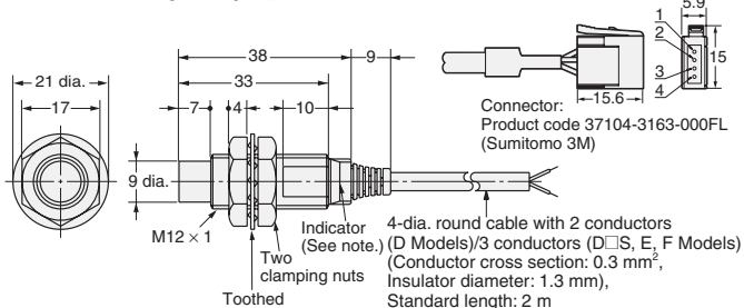
Fig. 9 : E2E-X8MD□ E2E-X5ME□/F□
