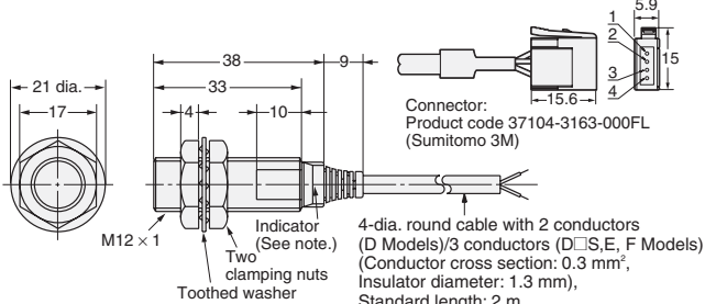
Fig. 8 : E2E-X3D□-N E2E-X2E□/F□
