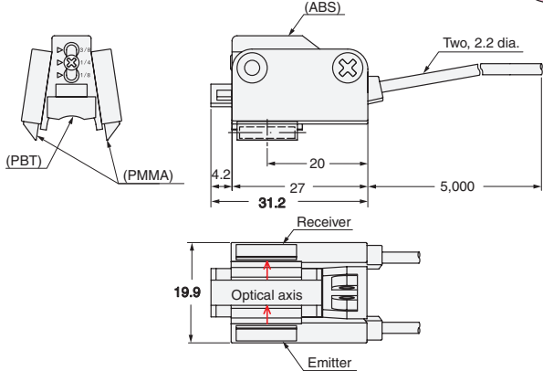
E32-D82F1 (R40) E32-D82F2 (R40)
