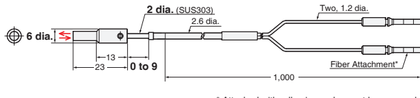
21-A E32-C42 1M (No Cutting) + E39-F3A
