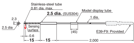
17-B E32-T24E 2M (Free Cutting)
