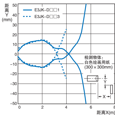
E3JK-D□□1/D□□3
