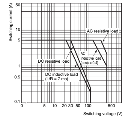
G2R-1Z, G2R-1AZ
