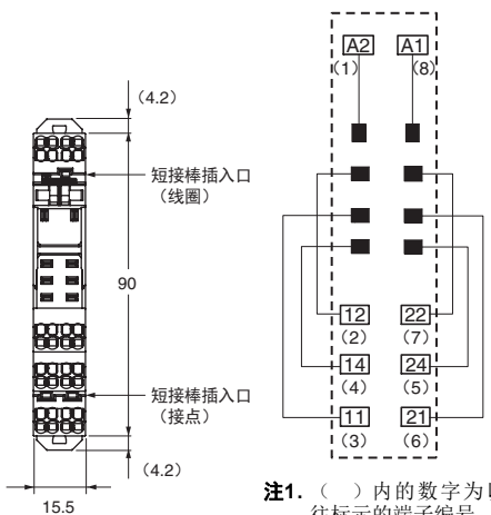
端子配置/内部连接图 (顶视图)
