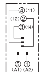
端子配置/内部连接图 (顶视图)
