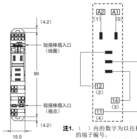
端子配置/内部连接图 (顶视图)
