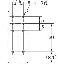
安装孔加工尺寸 (底视图)
