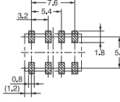
印刷基板加工尺寸 (BOTTOM VIEW) 尺寸公差±0.1mm
