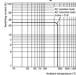
G7L-2A-T (TJ) (TUBJ) G7L-2A-B (BJ) (BUBJ) (BUBJ) Maximum Switching Power
