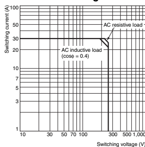
G7L-1A-T (TJ) (TUBJ) G7L-1A-B (BJ) (BUBJ) (BUBJ) Maximum Switching Power
