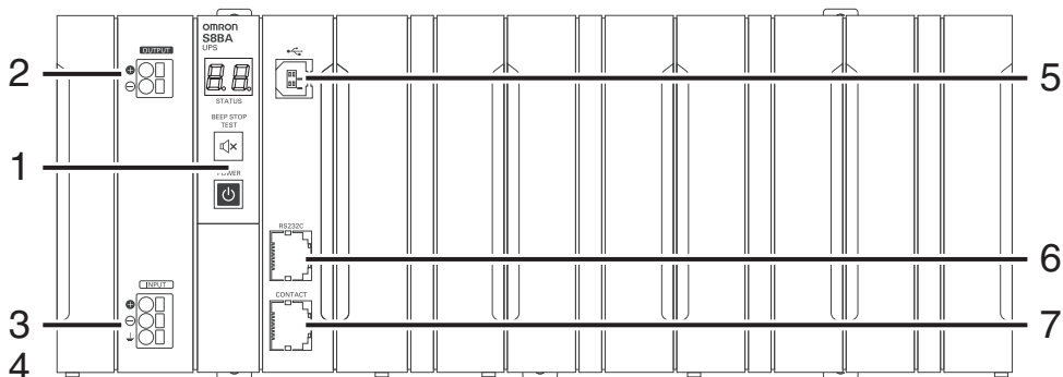
S8BA-24D24D480LF (480 W)
