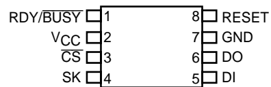
TSSOP Package (UR, YR)
