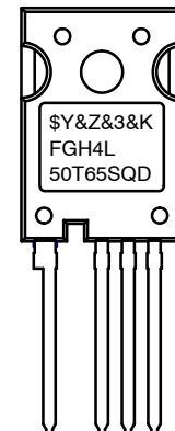
TO-247-4LD CASE 340CJ
