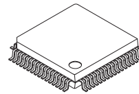
PQFP64 14x14 / Q1P64E [LC75852E]
