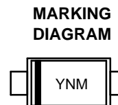
SOD-923 CASE 514AB
