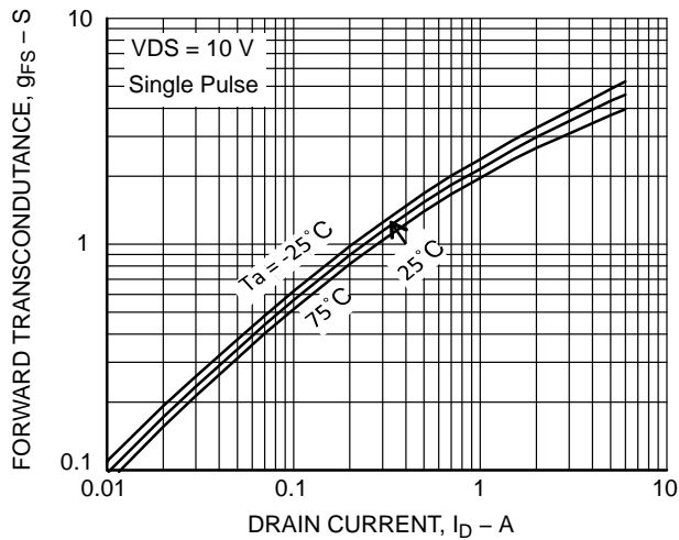
Figure 6. g_{FS} - I_D
