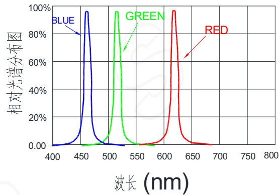
波长特性
