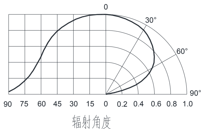
典型的辐射方向图 120^{\circ}
