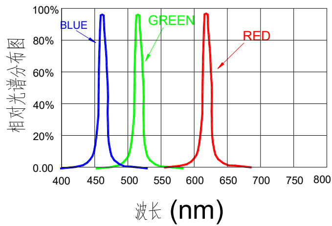
波长特性
