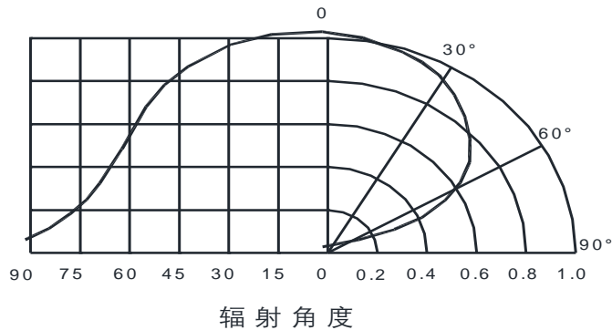
典型的辐射方向图 120°
