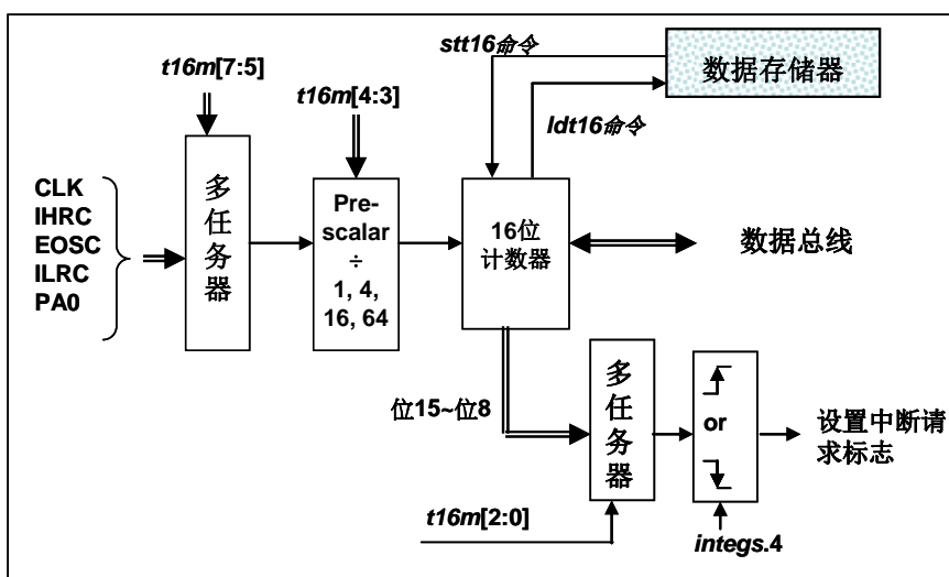
图 10: Timer16 模块框图
