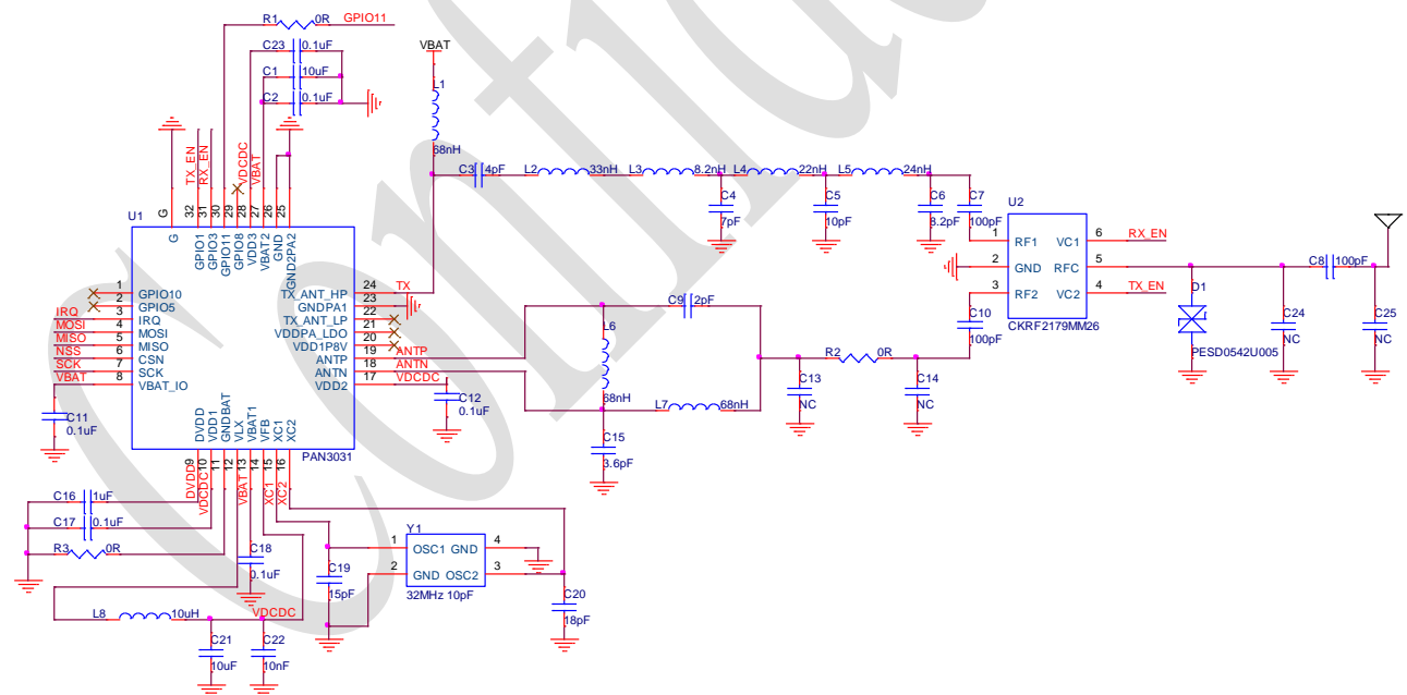
图 6-2 PAN3031 参考原理图（内部 DCDC 供电）
