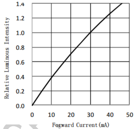
正向电流与相对光强特性曲线
