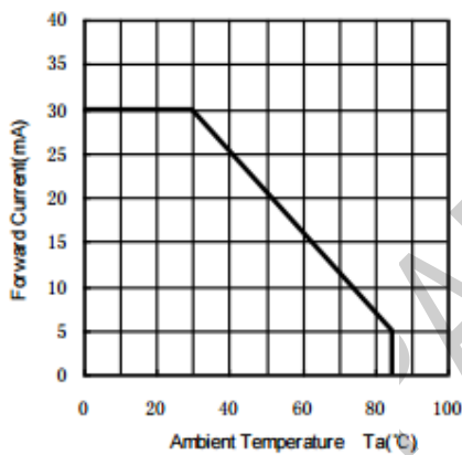
环境温度与正向电流特性曲线
