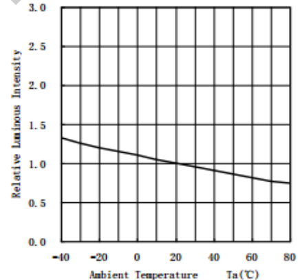
环境温度与相对光强特性曲线
