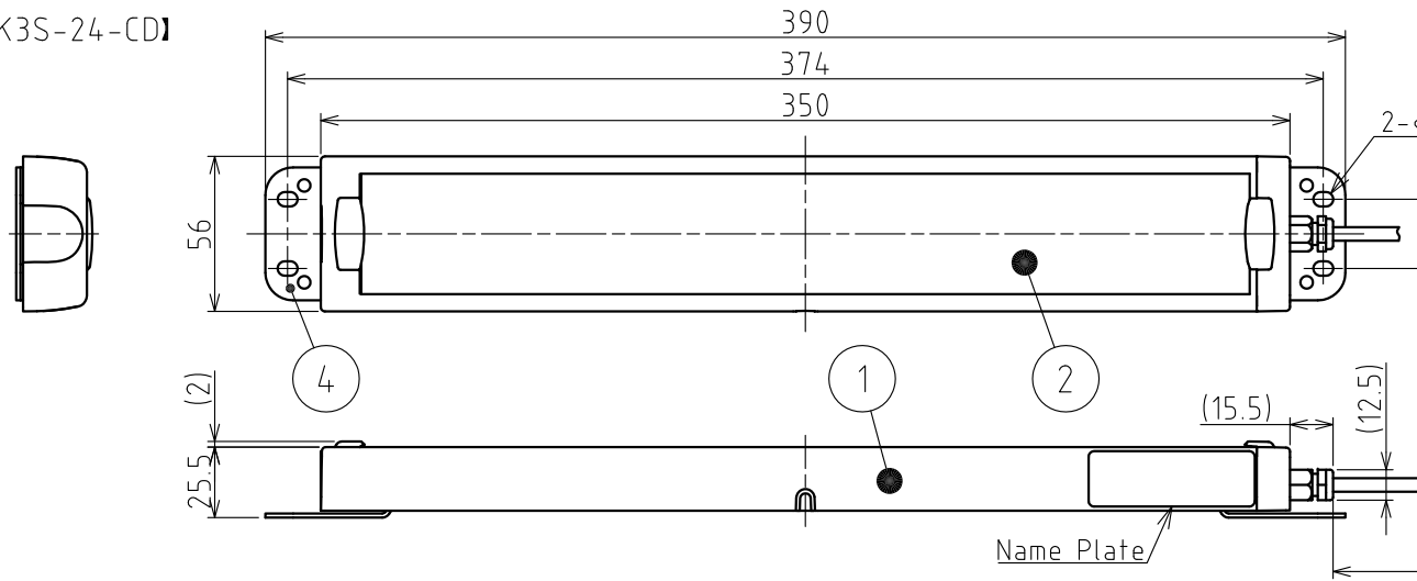
【CWK6S-24-CD】
