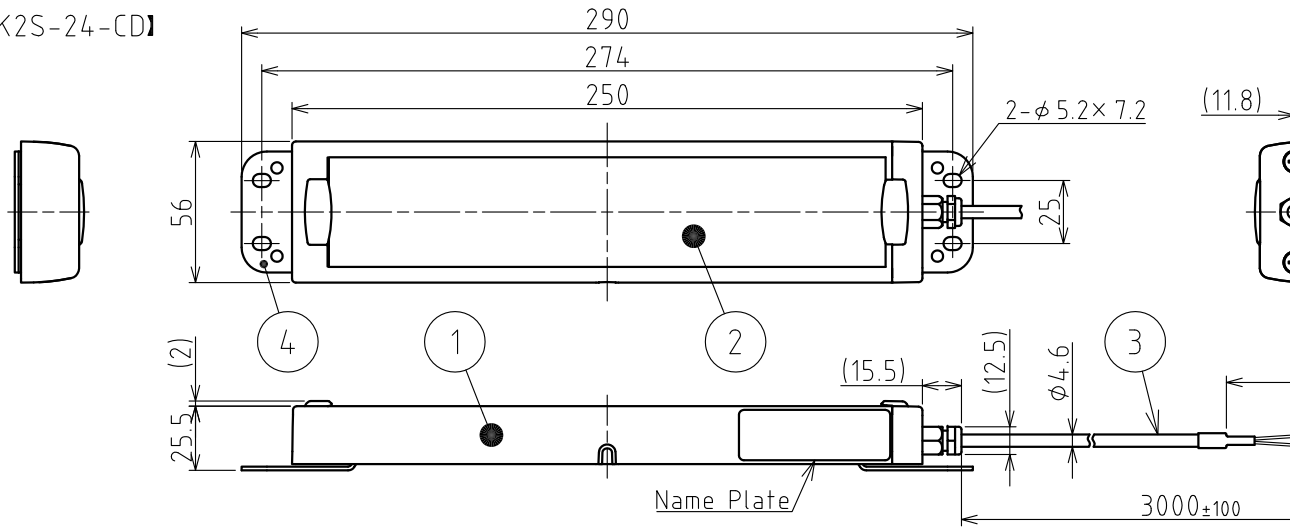
【CWK3S-24-CD】
