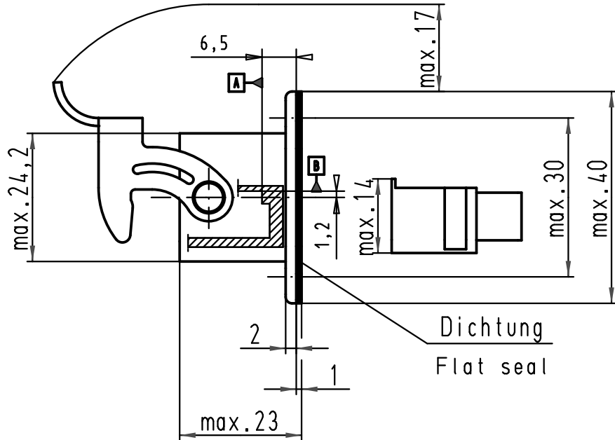
Zusammenbau assembly
