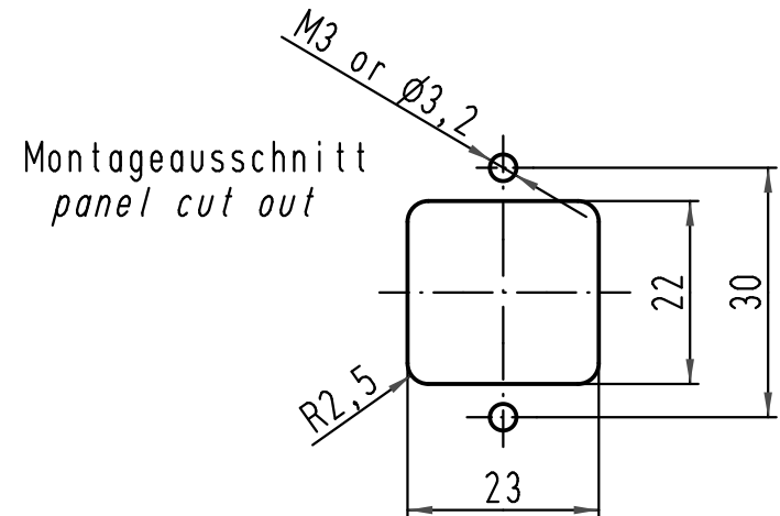
Metallgehäuse/metal housing
