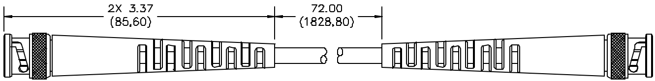
TRUE 75 BNC CABLE, RED (MODEL 6510-V-72-2)
