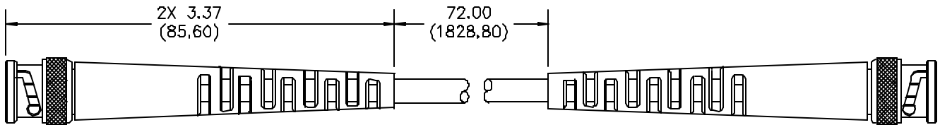
TRUE 75 BNC CABLE, BLUE (MODEL 6510-V-72-6)
