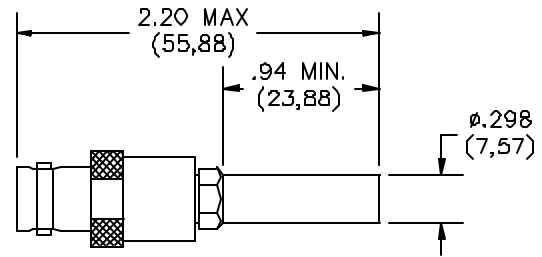
MINI WECO/BNC ADAPTER (4X MODEL 6519)
