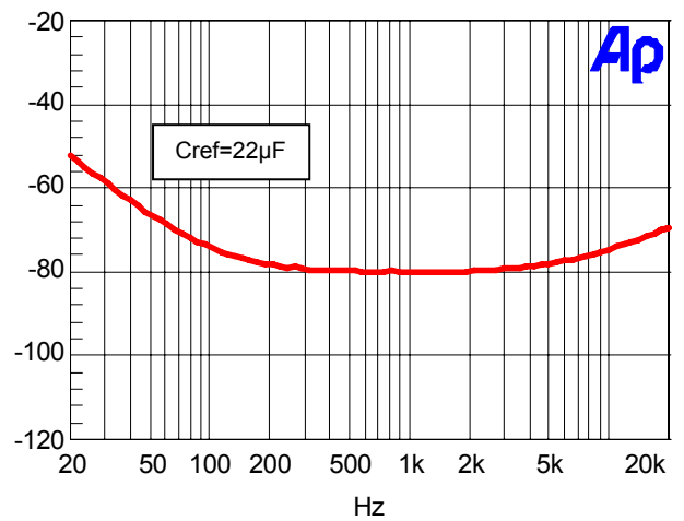
PSRR
