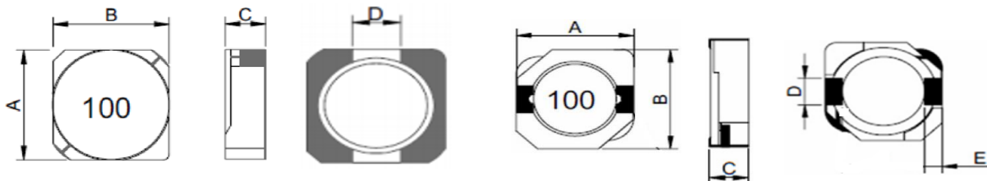
PSPHAQ4D18~6D38 尺寸图
