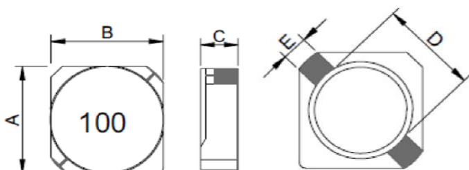
PSPHAQ2D11~3D28尺寸图
