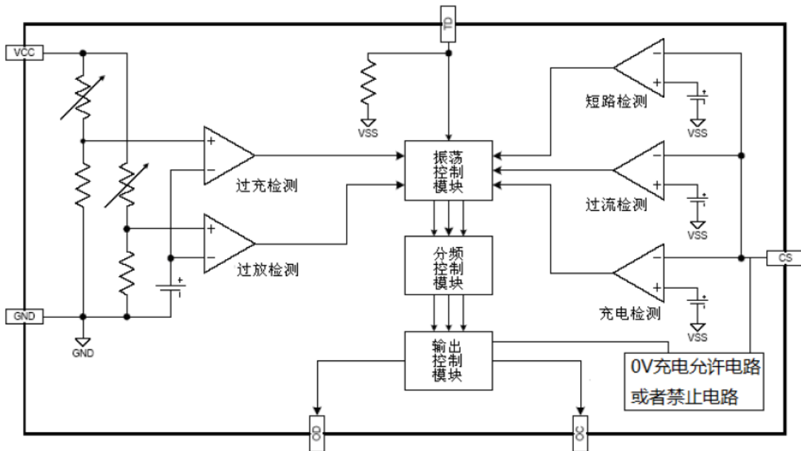
系统框图
