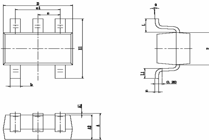
SOT353
