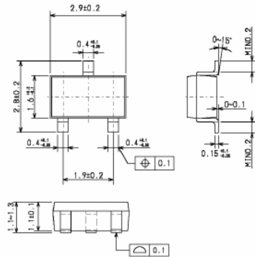
SOT23-3/SOT23-3B
